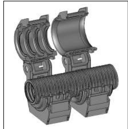
Hälfte des Federhalters Half of Spring Holder NW23/29: POFHB-23/29
