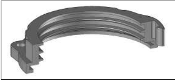
Hälfte der geraden Anschlussarmatur Half of Straight Connector NW70: PAGOB/G-70
