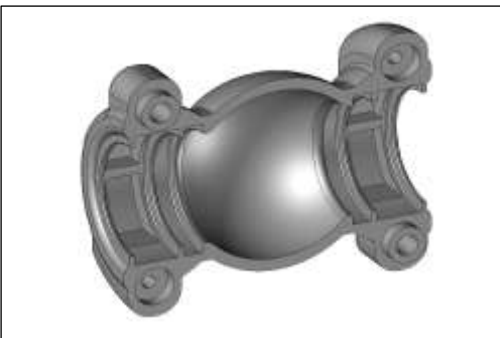
Hälfte des Verbindungsgelenkes Half of Connecting Joint NW23: PAVGB-23
