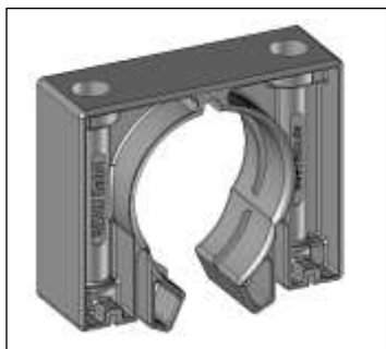
Verstärkter Systemhalter Strengthened System Support NW48: VPHOB-48
