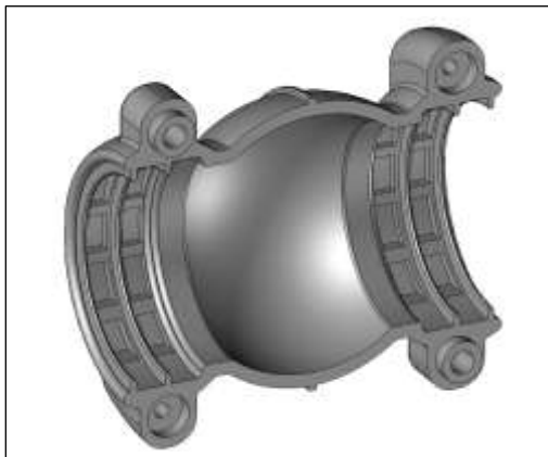
Hälfte des Verbindungsgelenkes Half of Connecting Joint NW36: PAVGB-36
