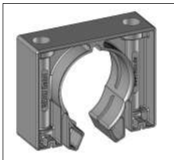
Verstärkter Systemhalter Strengthened System Support NW29: VPHOB-29
